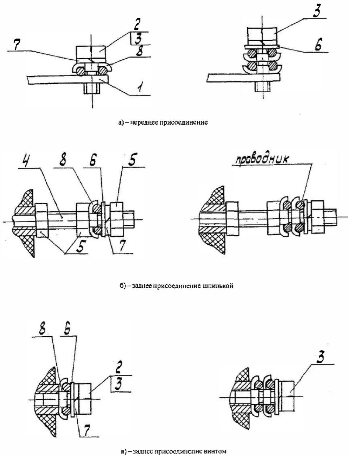
Рисунок 4 – Подсоединение внешних проводников
