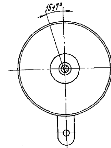
Рисунок 5 – Положение лыски при заведенном механизме времени
